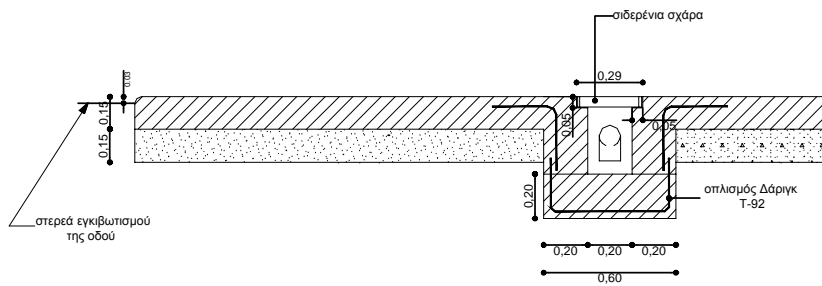
ΤΟΜΗ Β.1-Β.1
