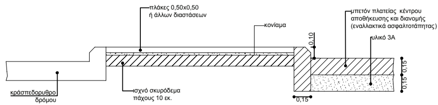
ΤΟΜΗ Α.1-Α.1
