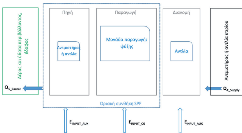
Σχήμα 1: Απεικόνιση των οριακών συνθηκών SPF για μονάδα παραγωγής ψύξης που χρησιμοποιεί τυπικό SPF και τηλεψύξη (και άλλα μεγάλα συστήματα ψύξης που χρησιμοποιούν μετρούμενο SPF), όπου « E_{INPUT\_AUX} » είναι η εισροή ενέργειας στον ανεμιστήρα και/ή στην αντλία και « E_{INPUT\_CG} » η εισροή ενέργειας στη μονάδα παραγωγής ψύξης.
