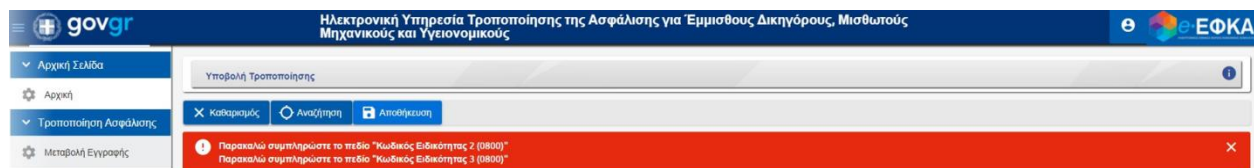
Εικόνα 2 Μήνυμα Σφάλματος 2
