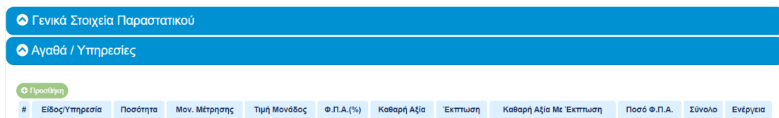
Εικόνα 6. Αναδίπλωση επιλογών
